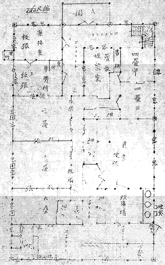
圖面平階一
